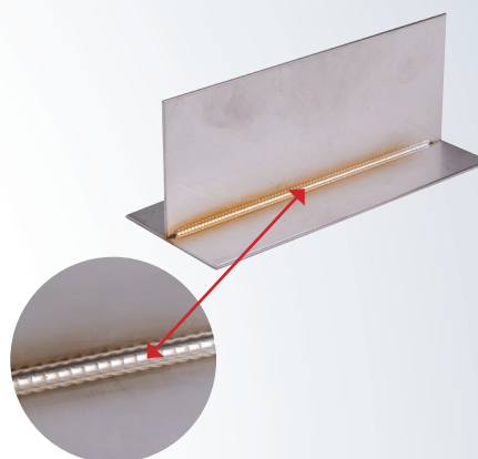
Sarok ponthegeesztés 0,6 mm vastagság
