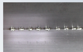
Sarok ponthegeesztés 0,6 mm vastagság
